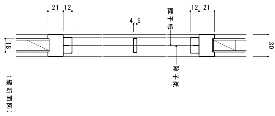
【3 御殿襖 詳細図】
